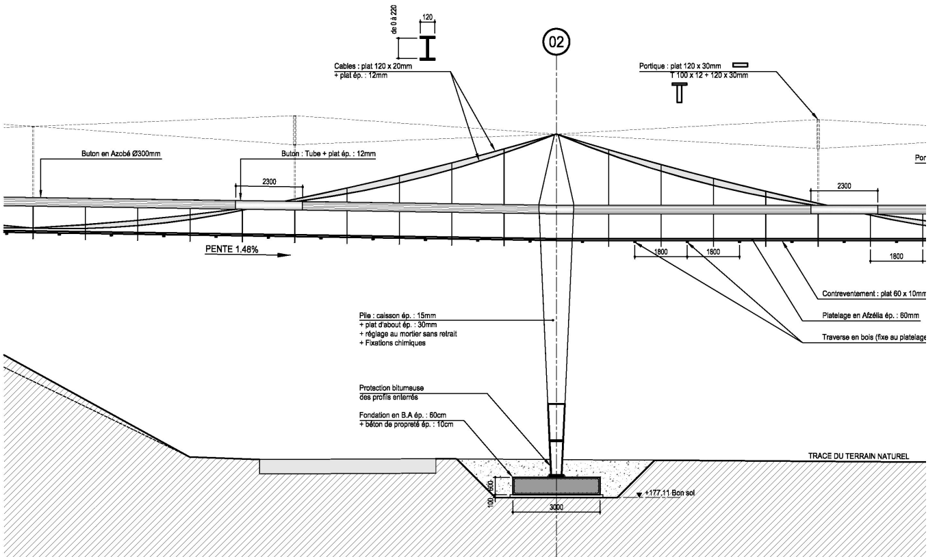
VUE EN ELEVATION PASSERELLE (2007 - 11/06)
